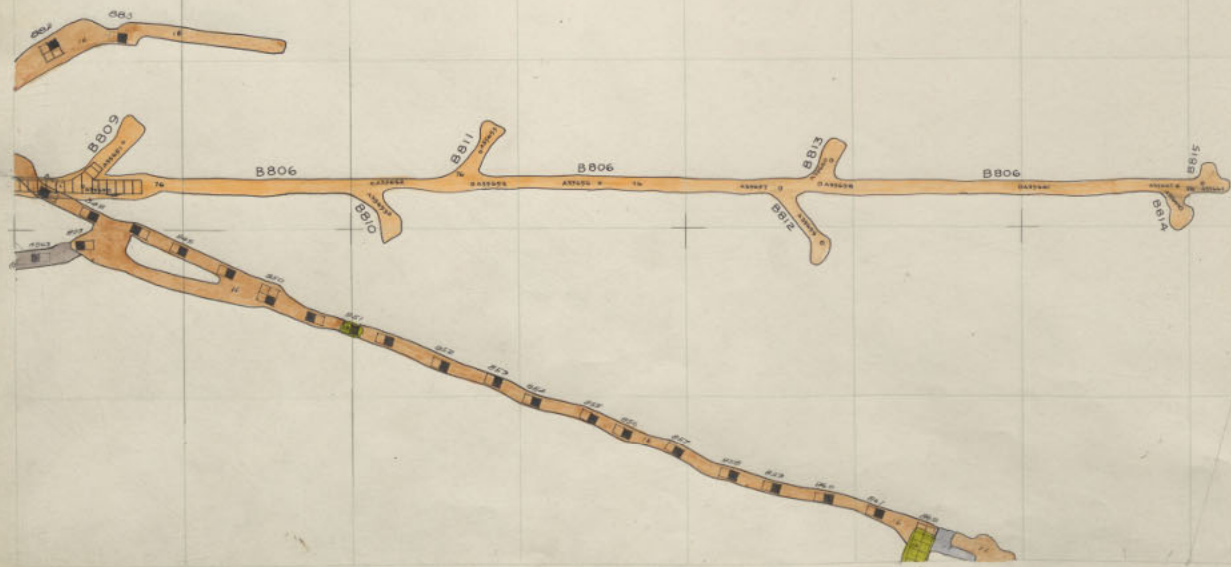
Berkeley 800-10. ELEV. 4999 " (TUNNEL) 800 - SILL
